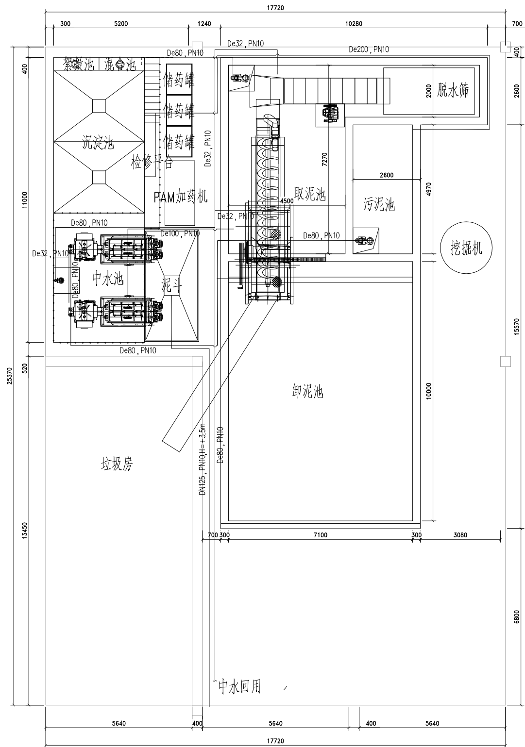
总平面布置图
